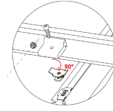
Dispositif anti-glisement pour le climber 63
