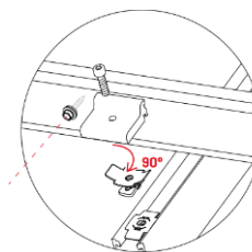
Dispositif anti-glisement pour climber 63
